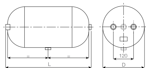
4 bosses M22x1,5
