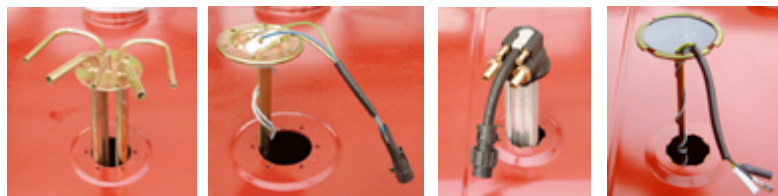
Pescanti e comandi indicatore livello su flangia 6 fori e su flangia dentellata
