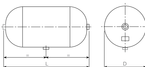
* 3 borchie M22x1,5
