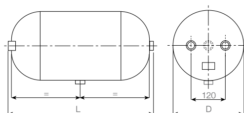
4 borchie M22x1,5
